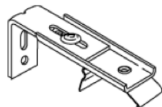
Produit : SV-92-29 Dim. : 2-7/8" @ 3-7/8" (73-98mm) Quantité par boîte : 250
