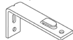
Produit : SV-36 Dimensions : 2.8" (71mm) Quantité par boîte : 400
