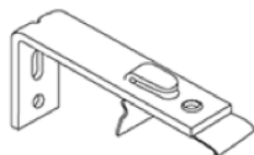
Produit : SV-40 Dimensions : 3-3/8" (85mm) Quantité par boîte : 400
