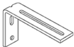
Produit : SV-30 Dimensions : 3-3/8" (85mm) Quantité par boîte : 350
