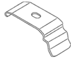
Produit : SV-4N Dimensions : 1-13/16" (56mm) Quantité par boîte : 1500 Type : Sunteca-Deco
