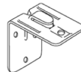
Produit : SV-7 Dimensions : 1-5/8" (41mm) Quantité par boîte : 500
