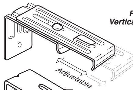
SV-52 100 per Box 1 1 / 8 " - 1 15 / 16 " (27 - 50mm)
